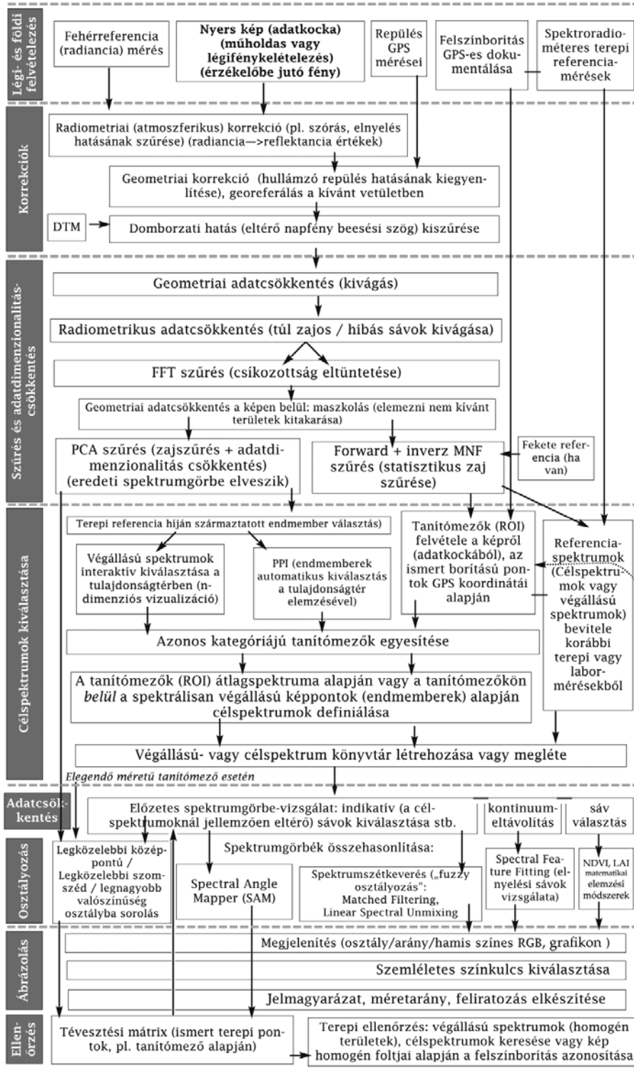
3. ábra: A hiperspektrális képek feldolgozásának vázlatja
