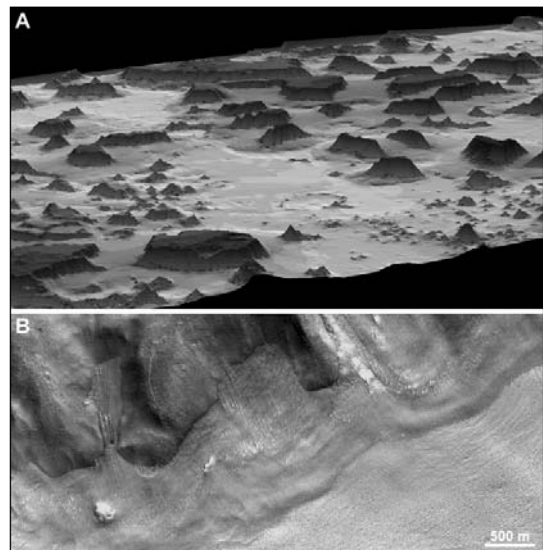
6. ábra A – a kimart területek jellemző relief-viszonyait ábrázoló digitális domborzatmodell (5-szörös magasságtorzítás); B – egy völgy oldalfala mentén húzódó törmelékletjtő képe az MGS MOC M0304315 számú nagyfelbontású felvételén
